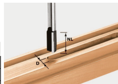
Schaft Ø 12 mm
